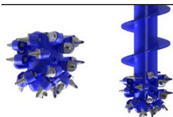
Głowica frezująca okrągłymi nożami oraz nożami typu Dragontooth
